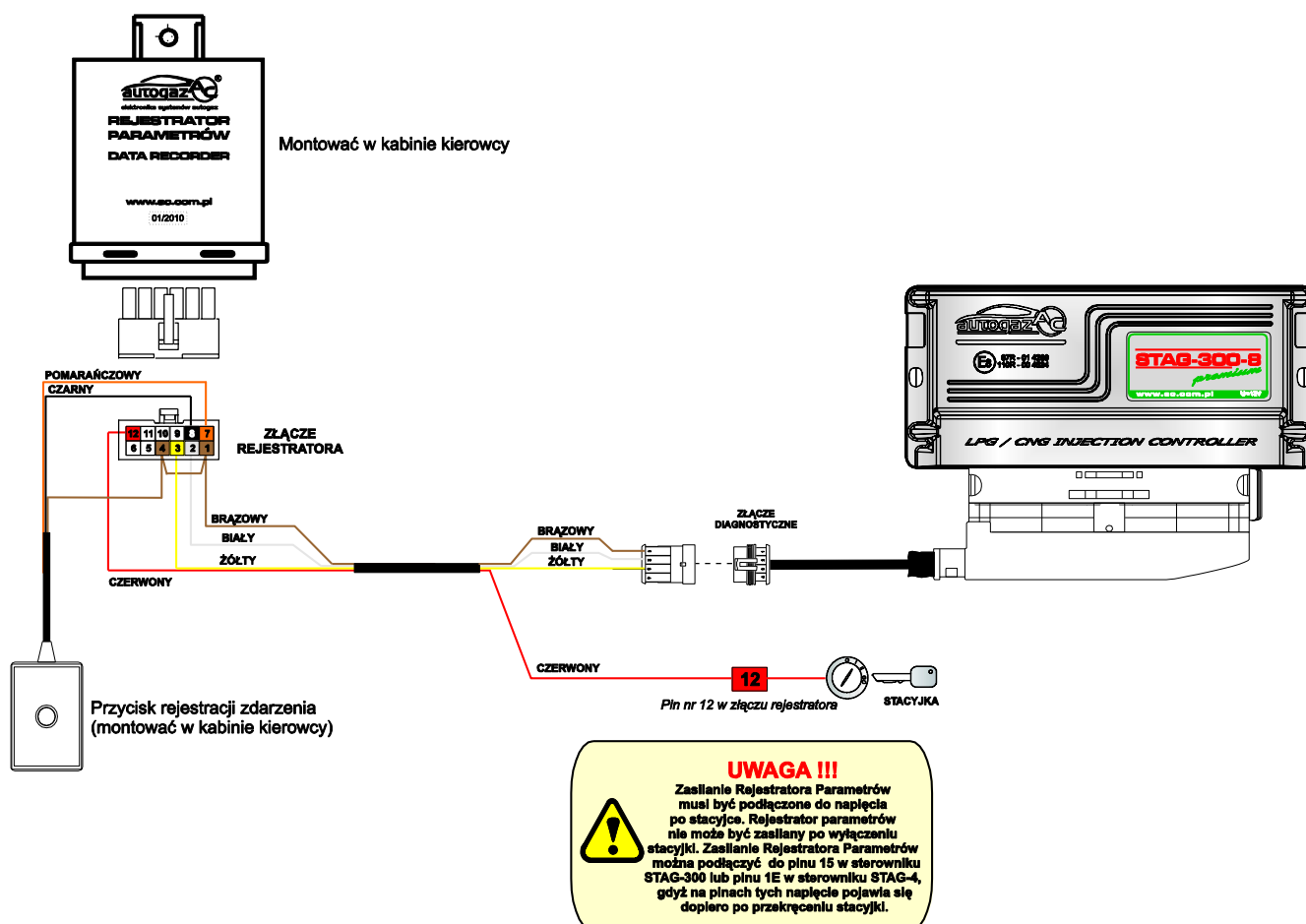
Rysunek 1. Schemat podłączenia Rejestratora Parametrów do instalacji samochodu.
