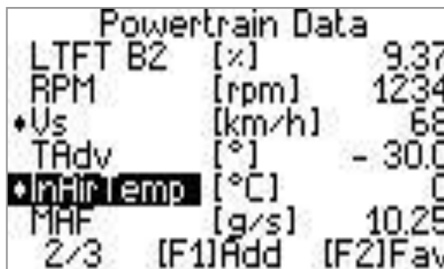
Fig 2.4.2: Powertrain Data box
