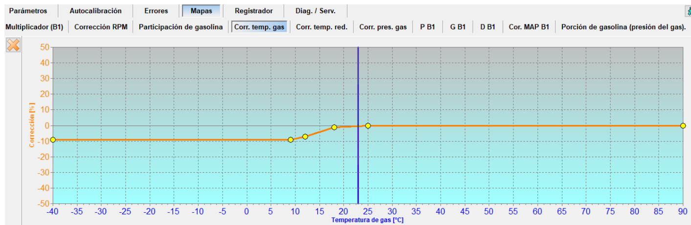
Figura 37 Mapa "Corrección de la temperatura del gas"
