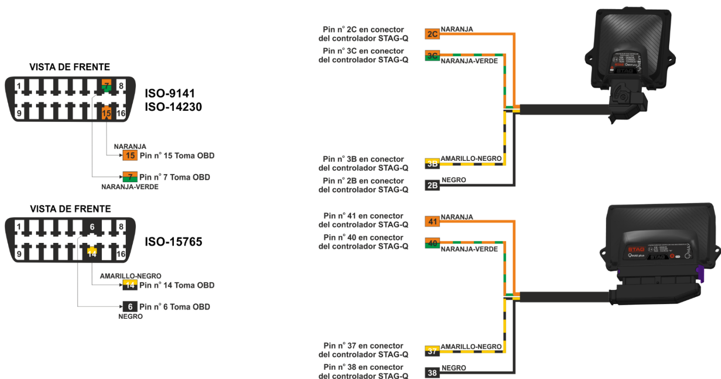
Figura 5 Esquema de conexión STAG: QNEXT PLUS / QMAX PLUS al enchufe OBD.
