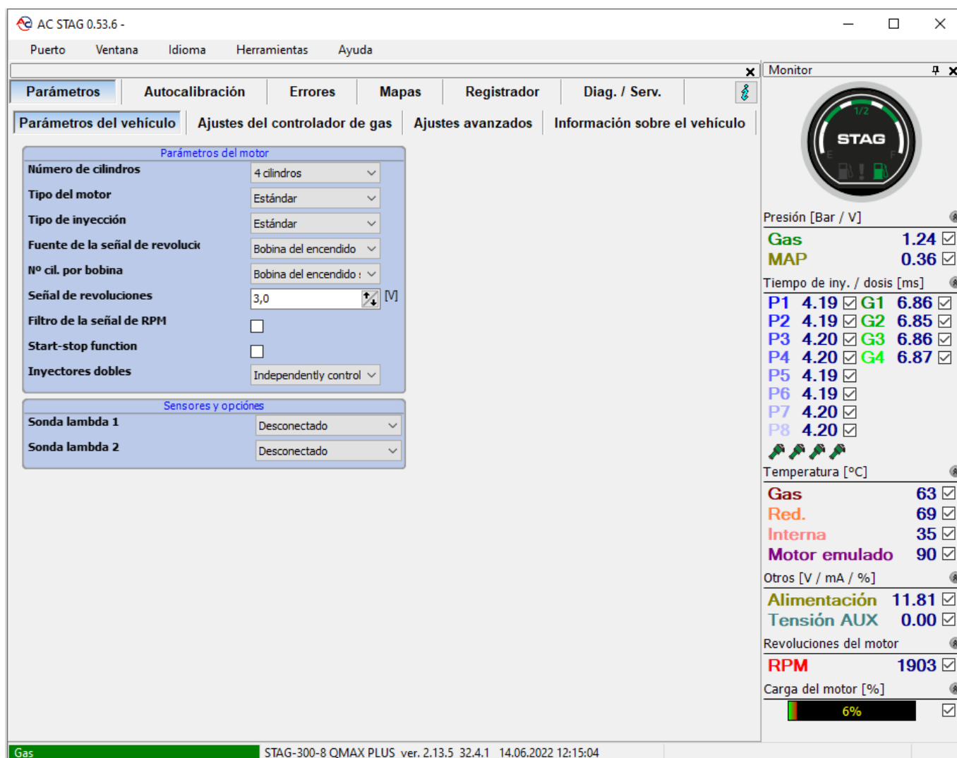
Figura 17 Vista de la configuración de los inyectores dobles controlados individualmente
