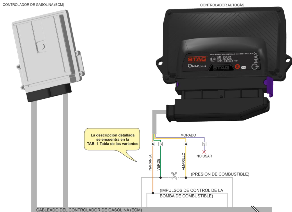
Figura 7 Esquema de conexión Emulador de presión de combustible FPE en STAG-300 QMAX PLUS.
