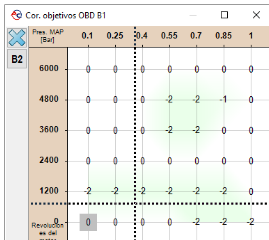
Figura 53 Mapa de las correcciones OBD de destino.
