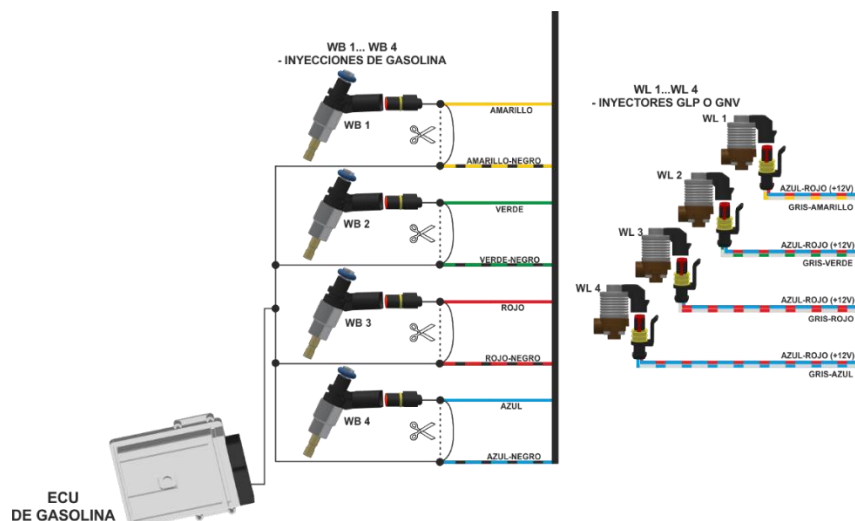
Figura 9 Esquema de conexión a la instalación del vehículo con el control full group..
