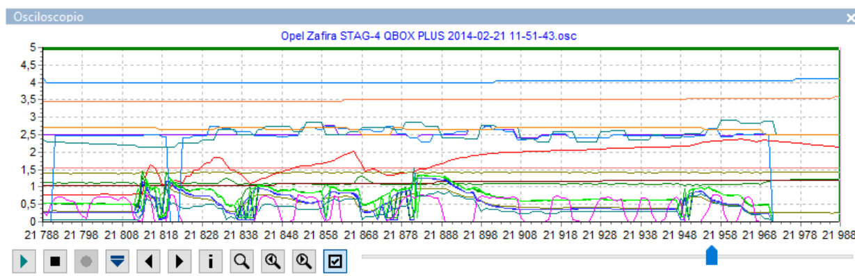
Figura 25 Vista del osciloscopio
