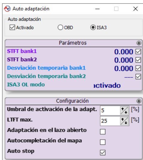
Figura 51 Configuración de la adaptación ISA3
