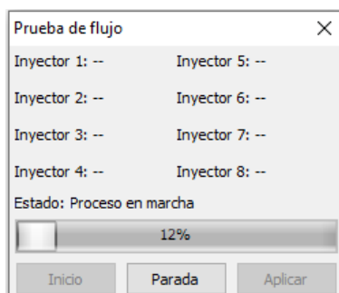
Figura 21 Prueba de caudal de los inyectores de gas
