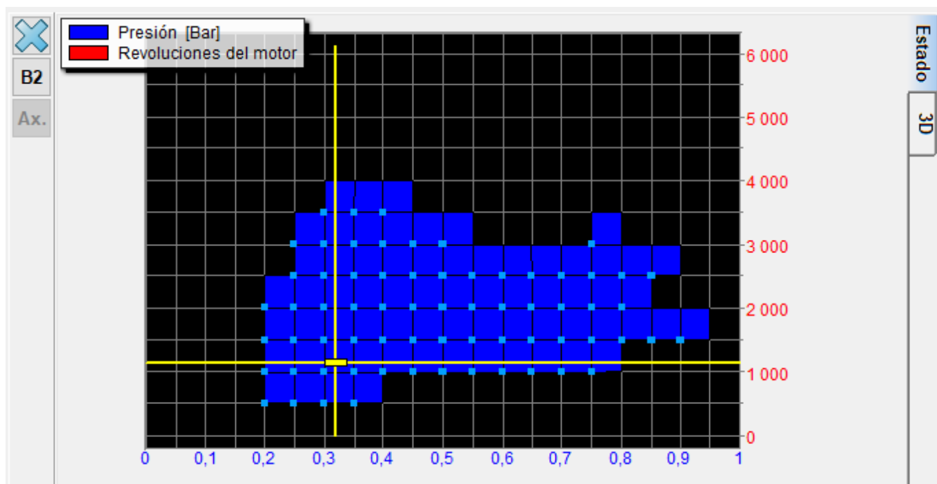
Figura 42 Estado de recogida del mapa de gasolina
