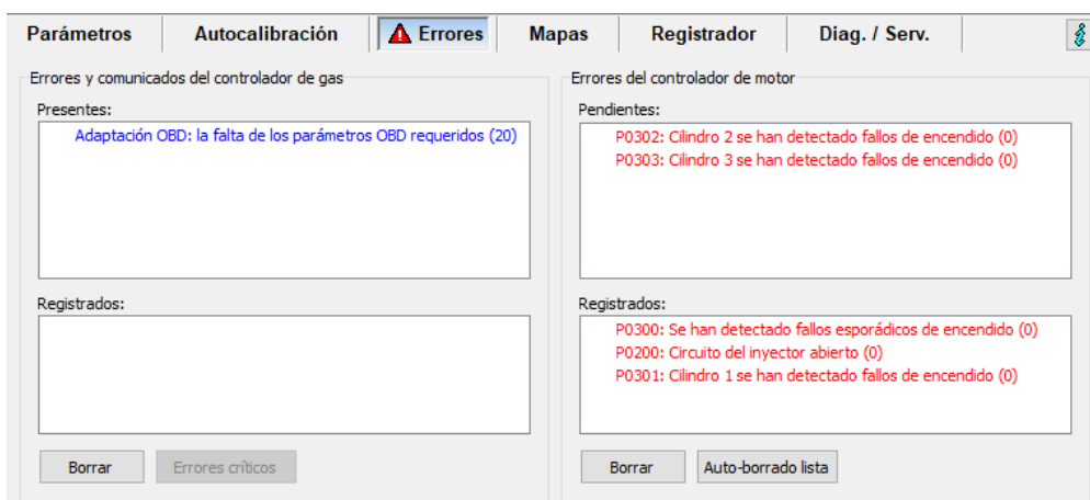
Figura 28 Vista de la pestaña errores. Defectos OBD
