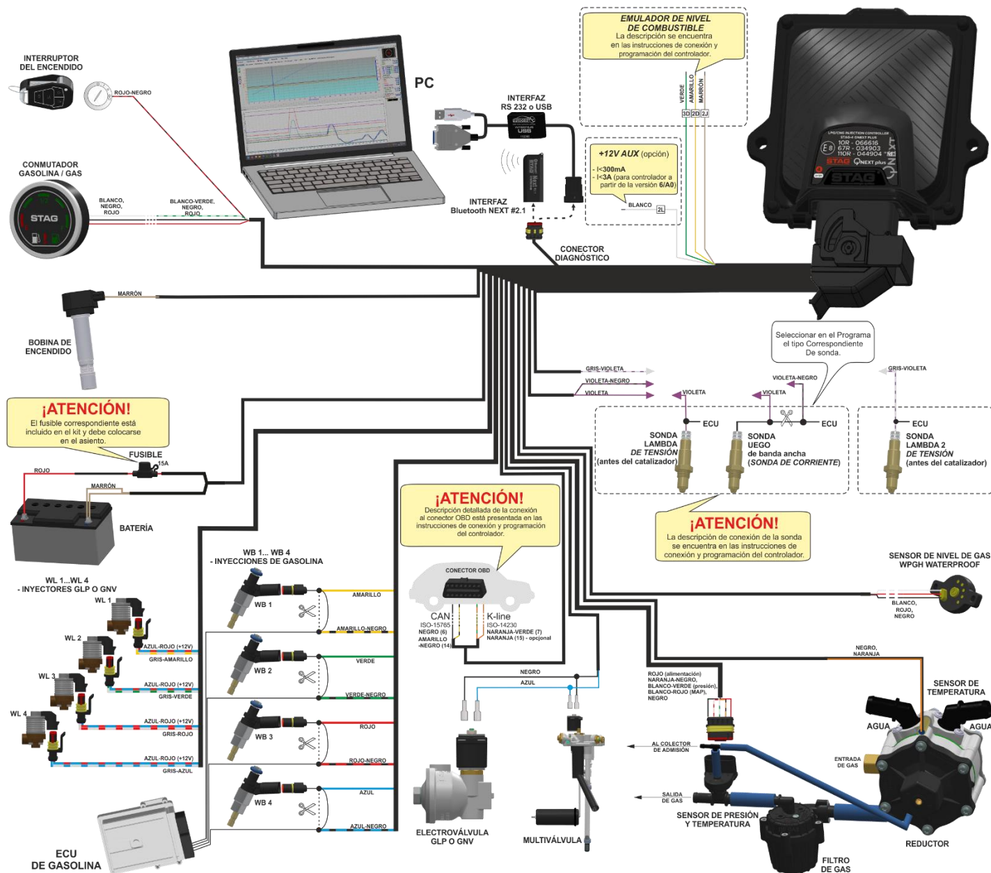
Figura 2 Esquema de conexión STAG-4 QNEXT PLUS a la instalación del vehículo.
