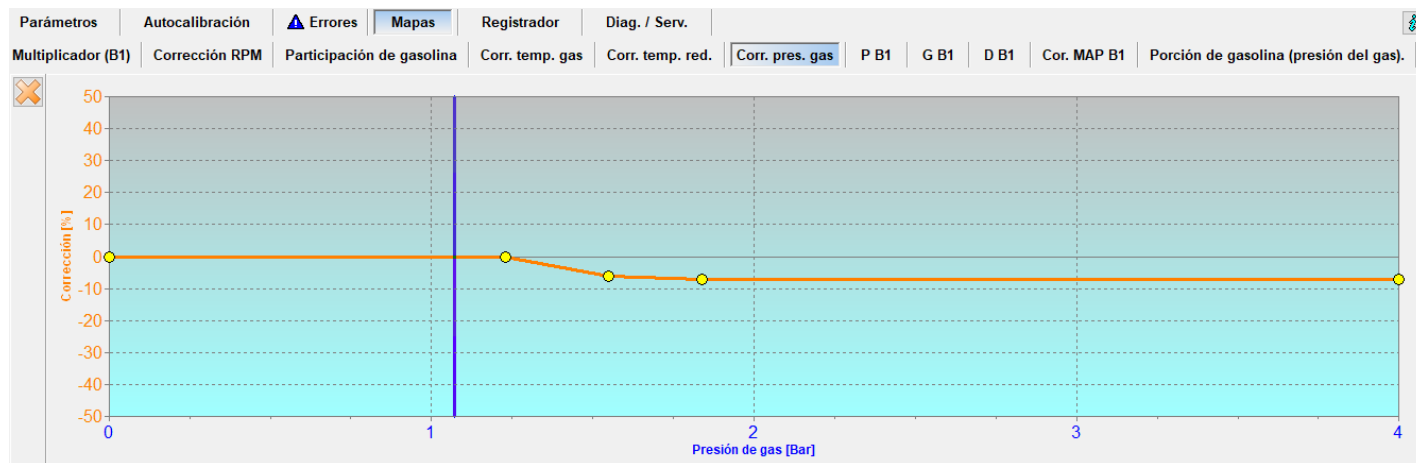
Figura 39 Mapa "Corrección de la presión del gas"
