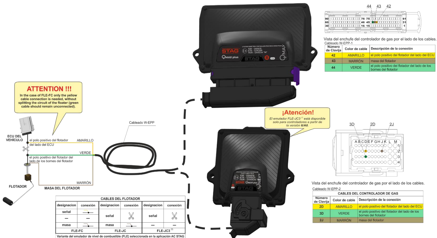
Figura 6 Esquema de conexión Emulador del nivel de combustible FLE en STAG: QNEXT PLUS / QMAX PLUS.
