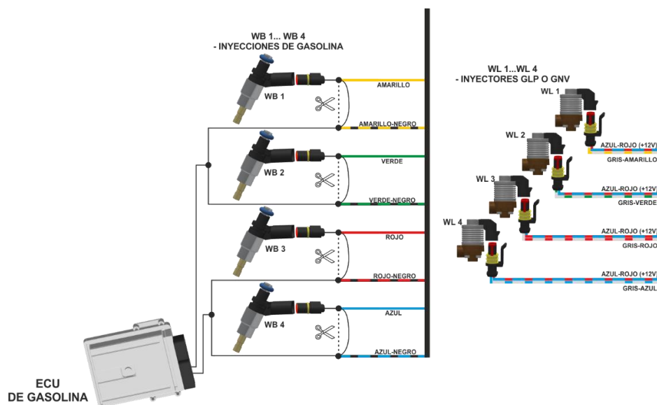
Figura 8 Esquema de conexión a la instalación del vehículo con el control semi-secuencial.
