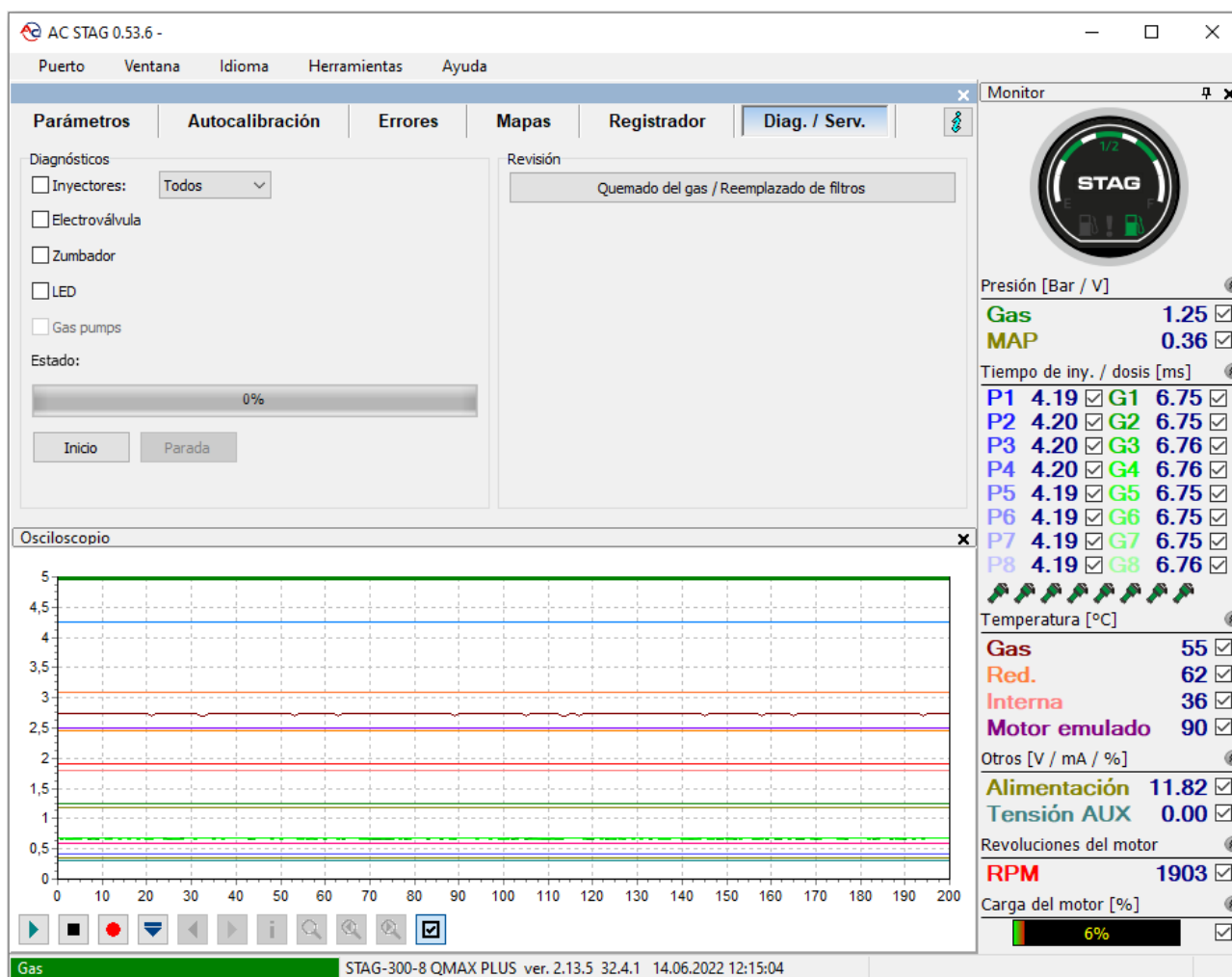
Figura 54 Vista de la ventana de Diagnóstico / servicio
