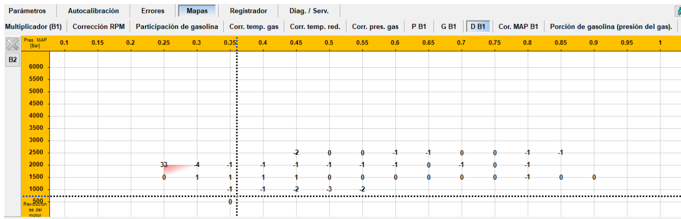
Figura 44 Mapa de desviación D
