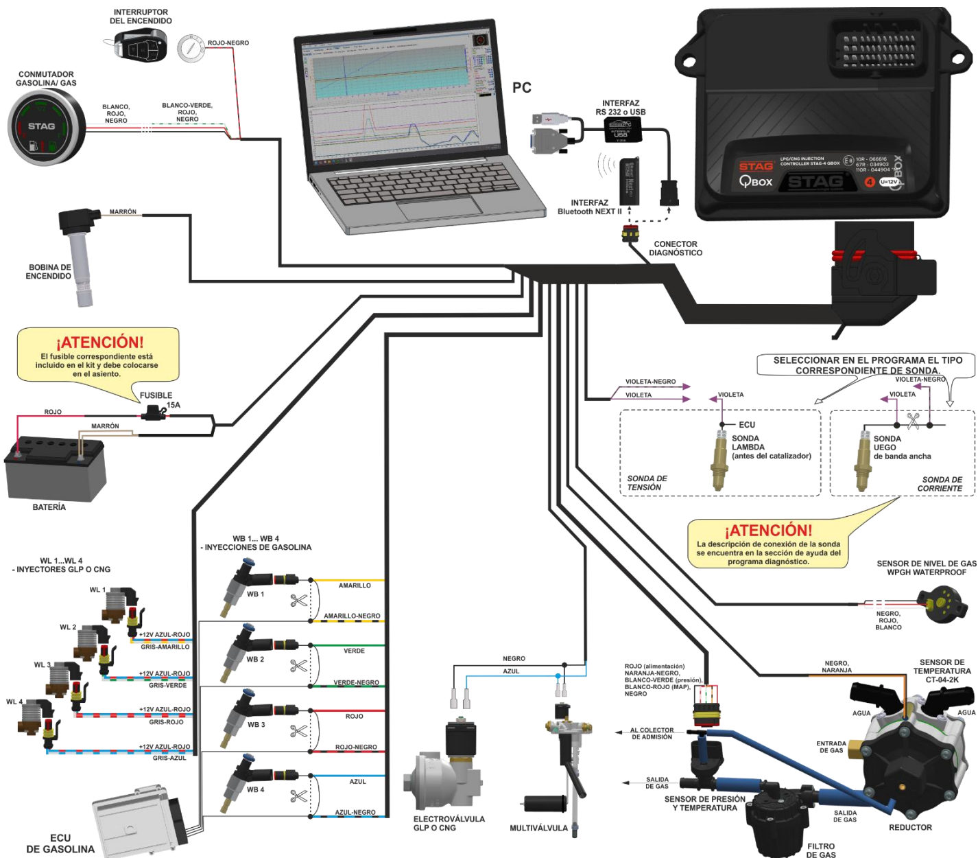
Figura 1 Esquema de conexión STAG-4 QBOX a la instalación del vehículo.
