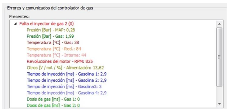
Figura 27 Marco „congelado” del error del inyector
