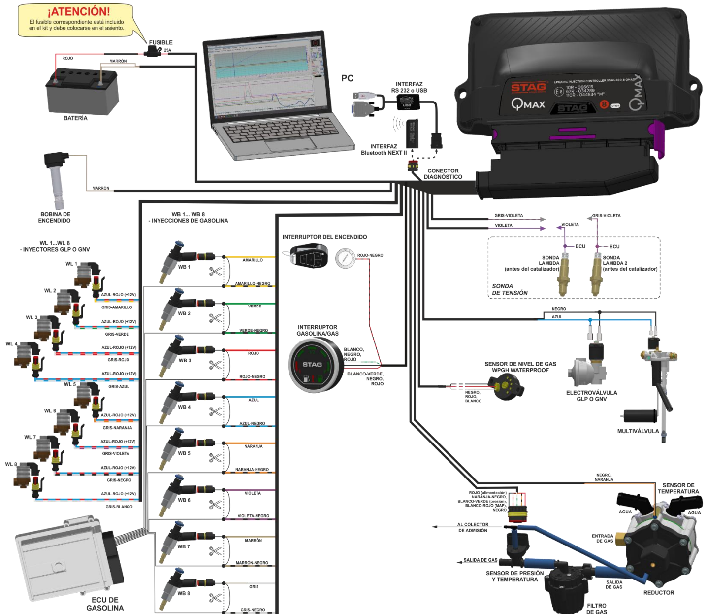
Figura 3 Esquema de conexión STAG-300 QMAX a la instalación del vehículo.
