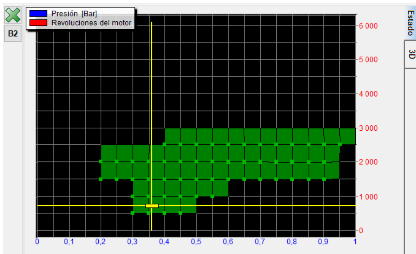
Figura 43 Estado de recogida del mapa de gas
