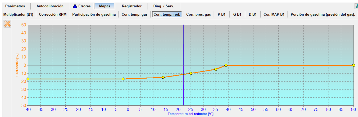
Figura 38 Mapa "Corrección de la temperatura del reductor"
