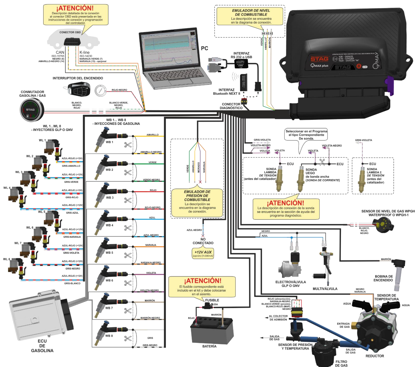
Figura 4 Esquema de conexión STAG-300 QMAX PLUS a la instalación del vehículo.
