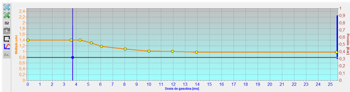
Figura 31 Mapa del multiplicador. Zona sugerida de "recogida" del mapa de gasolina
