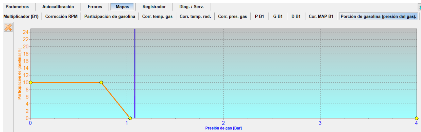
Figura 46 Mapa de proporción de gasolina (presión de gas)
