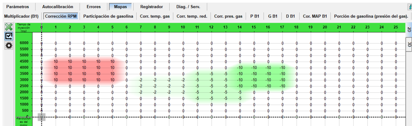
Figura 34 Vista del mapa de corrección de las revoluciones
