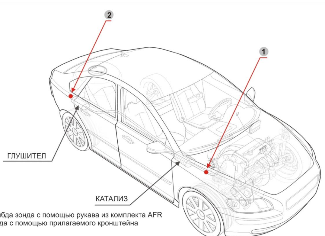
Рисунок 2 Место монтажа Лямбда-зонд
