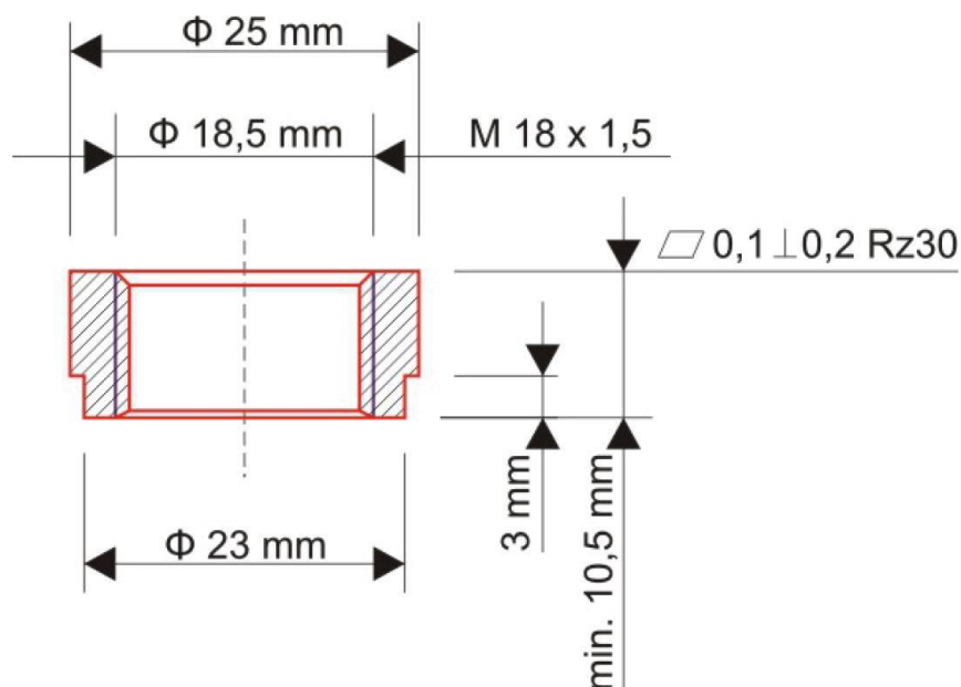
Рисунок 3 Рекомендованные размеры монтажной втулки лямбда-зонда
