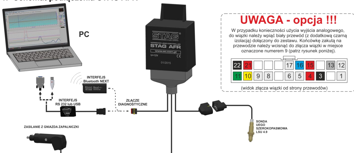
Rysunek 1 Schemat podłączenia
