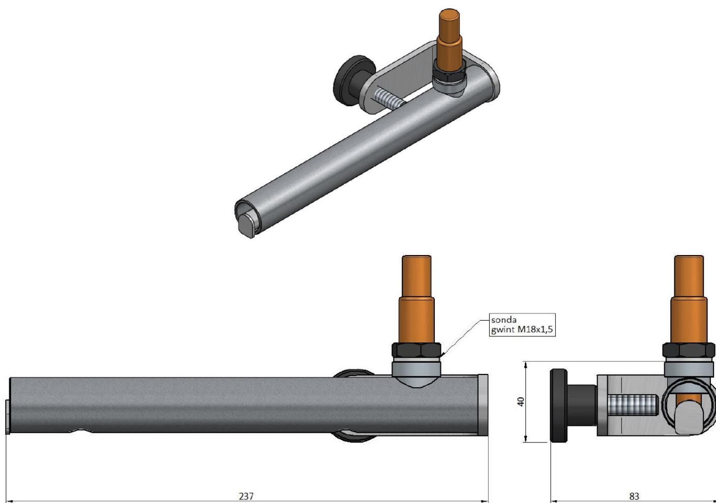
Rysunek 5 Prowadnica spalin z umieszczoną sondą.
