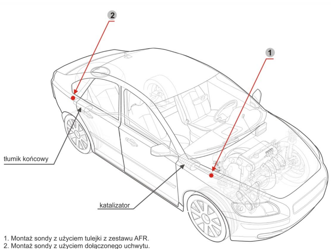
Rysunek 2 Miejsce montażu sondy Lambda
