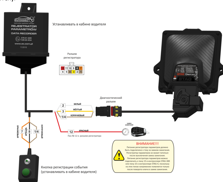
Рисунок 1. Схема подключения Регистратора параметров к установке автомобиля.
