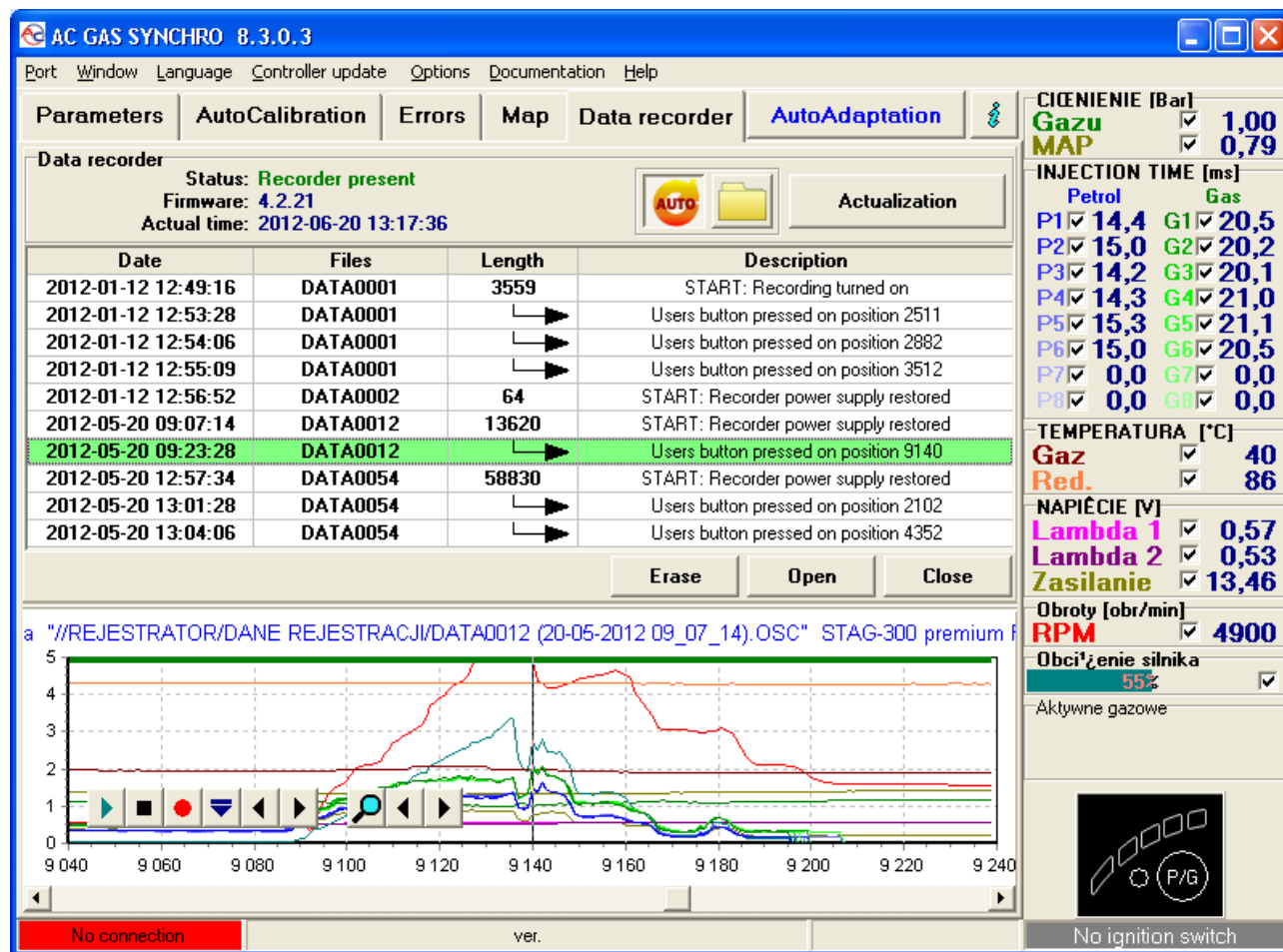
Fig. 2 Data recorder parameter window.
